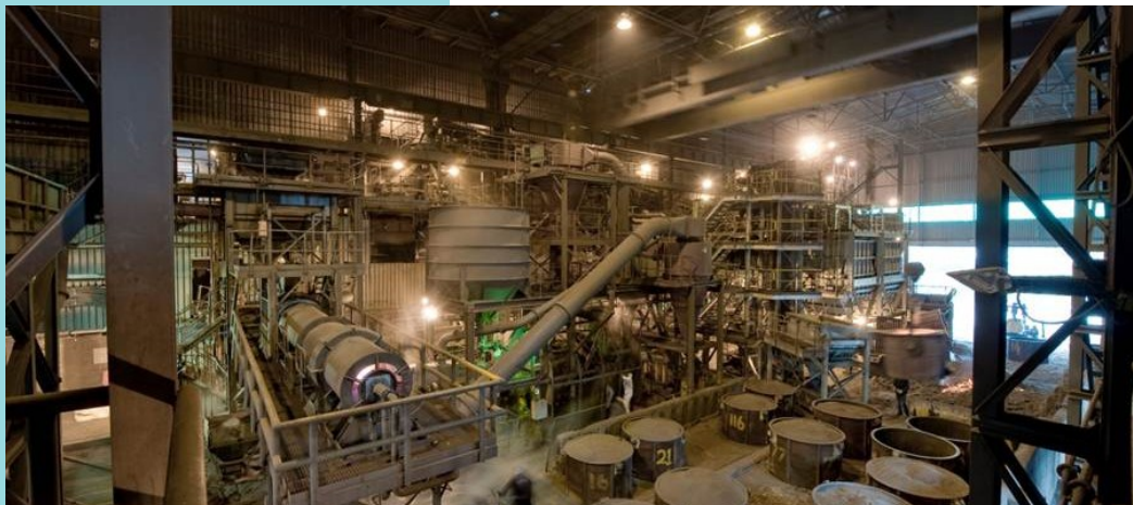
Завод DMS Powders в городе Мейертон, ЮАР
